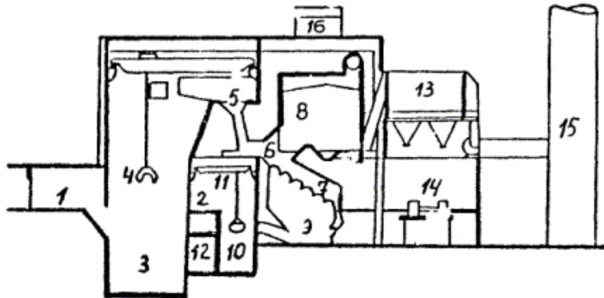
Рис. 1. Технологическая схема мусоросжигательного завода:
