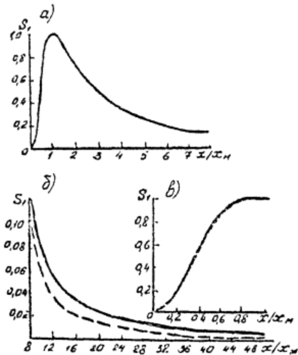
Рис. 6. График S = f(x/x_M) :
