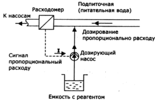
Рис. 1. Типовая схема дозирования
