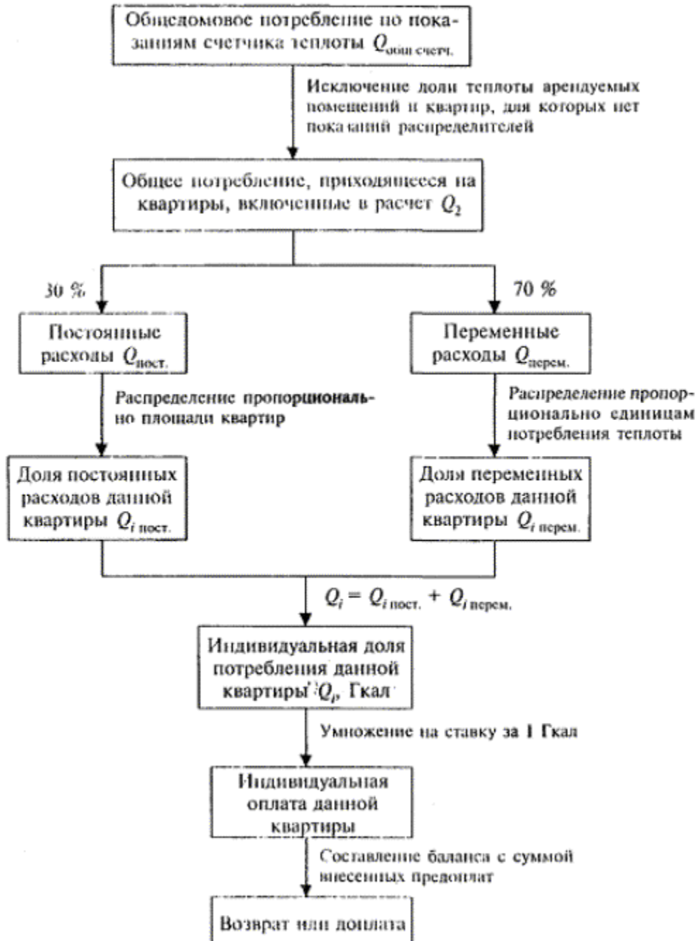
Рис 1. Обобщенная схема распределения общедомовых затрат тепловой энергии
